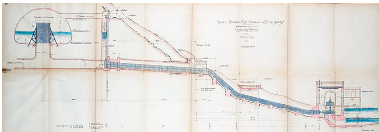
Forces motrices du Doubs. Usine hydro-électrique de Liebvillers [...] Ouvrages aval. Profil en long de l'ouvrage, octobre 1923.
