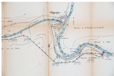
Forces motrices du Doubs. Usine Hydro-Électrique de Liebvillers. Plan sommaire des lieux et des ouvrages projetés [détail de Saint-Hippolyte], 1er novembre 1920 Phot. Jérôme Mongreville, Autr. Émile Andrié IVR43_20132500554NUCA4A
