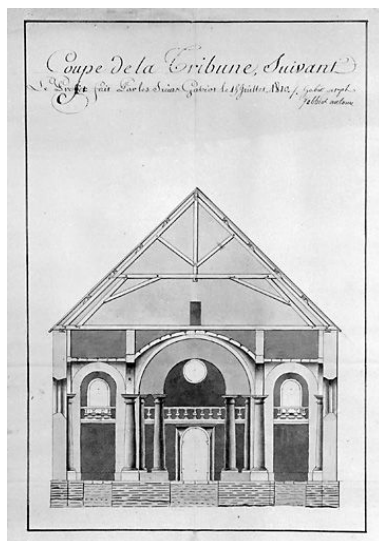
Coupe de la tribune, suivant le projet fait par les sieurs Gabiot le 15 juillet 1810. Dessin (plume, lavis), 1810, sans échelle. Phot. Jérôme Mongreville, Autr. Joseph (architecte) Gabiot, Autr. Antoine (architecte) Gabiot IVR43_19953900046X
