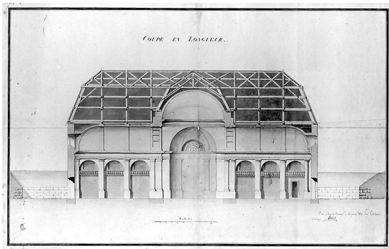
Coupe en longueur, 1813. Dessin (plume, lavis), 14 février 1813, échelle approximative 1:90.
