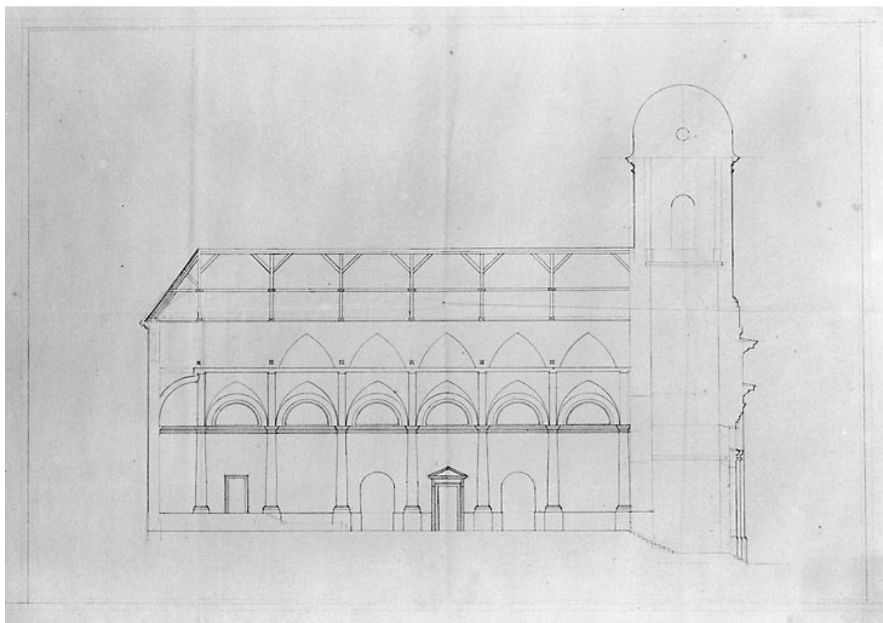
Coupe sur la longueur de l'église de Morez, 1810. Dessin (plume), s.d. [6 septembre 1810], sans échelle.
