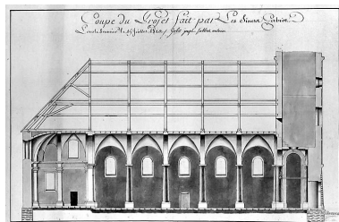
Coupe du projet fait par les sieurs Gabiot, 1810. Dessin (plume, lavis), 15 juillet 1810, sans échelle. Phot. Jérôme Mongreville, Autr. Joseph (architecte) Gabiot, Autr. Antoine (architecte) Gabiot IVR43_19953900003V
