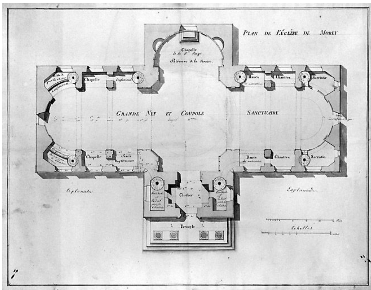
Plan de l'église de Morez, 1813. Dessin (plume, lavis), 14 février 1813, échelle approximative 1:90.
