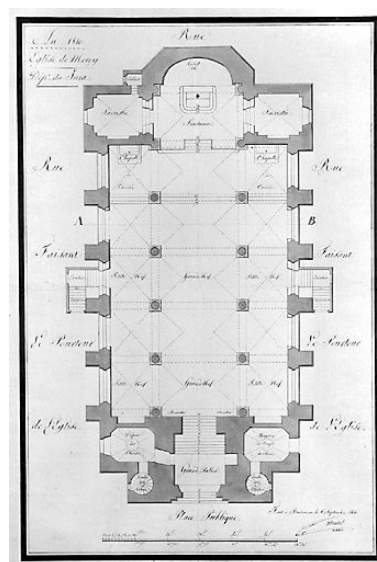
An 1810. Eglise de Morey [plan]. Dessin (plume, lavis), 6 septembre 1810, échelle approximative 1:100. Phot. Jérôme Mongreville, Autr. Claude-Antoine Colombot IVR43_19953900020V
