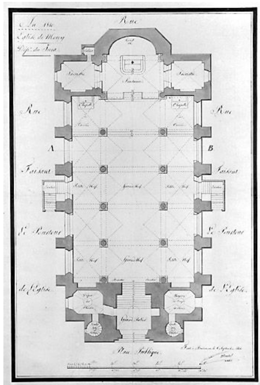
An 1810. Eglise de Morey [plan]. Dessin (plume, lavis), 6 septembre 1810, échelle approximative 1:100.
