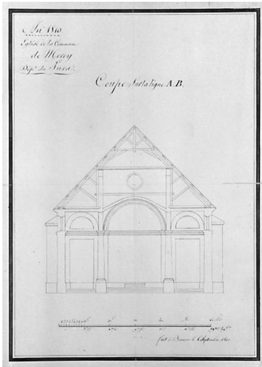
An 1810. Eglise de la commune de Morey. Coupe sur la ligne A.B. Dessin (plume), 6 septembre 1810, échelle approximative 1:100.
