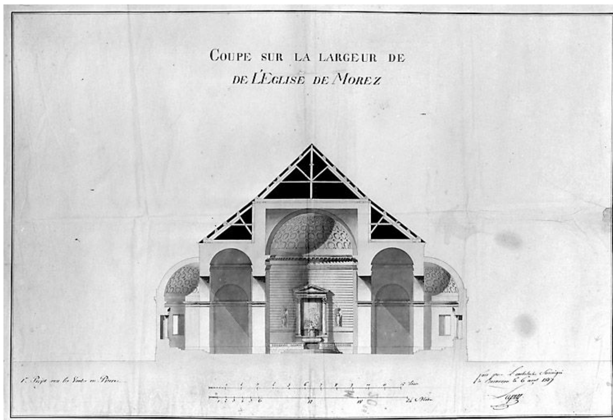
[Coupe sur la largeur de l'église de Morez], 1817. Dessin (plume, lavis), 6 août 1817, échelle approximative 1:120. Porte en note : 1er projet avec les voûtes en pierre.
