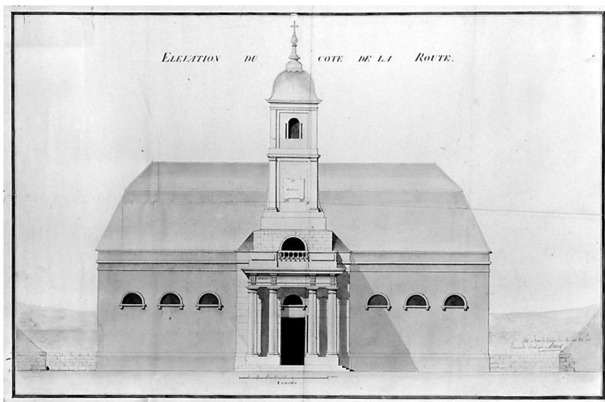
Elévation du côté de la route, 1813. Dessin (plume, lavis), 14 février 1813, échelle approximative 1:90.
