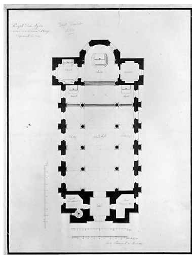
Projet d'une église à construire dans la commune de Morey, 1810. Dessin (plume, lavis), 14 mars 1810. Phot. Jérôme Mongreville, Autr. Claude-Antoine Colombot IVR43_19953900005V
