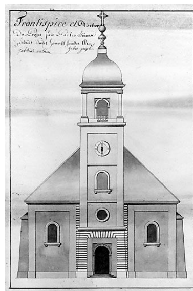
Frontispice et clocher du projet fait par les sieurs Gabiot dudit jour 15 juillet 1810. Dessin (plume, lavis), 1810, sans échelle. Phot. Jérôme Mongreville, Autr. Joseph (architecte) Gabiot, Autr. Antoine (architecte) Gabiot IVR43_19953900015V
