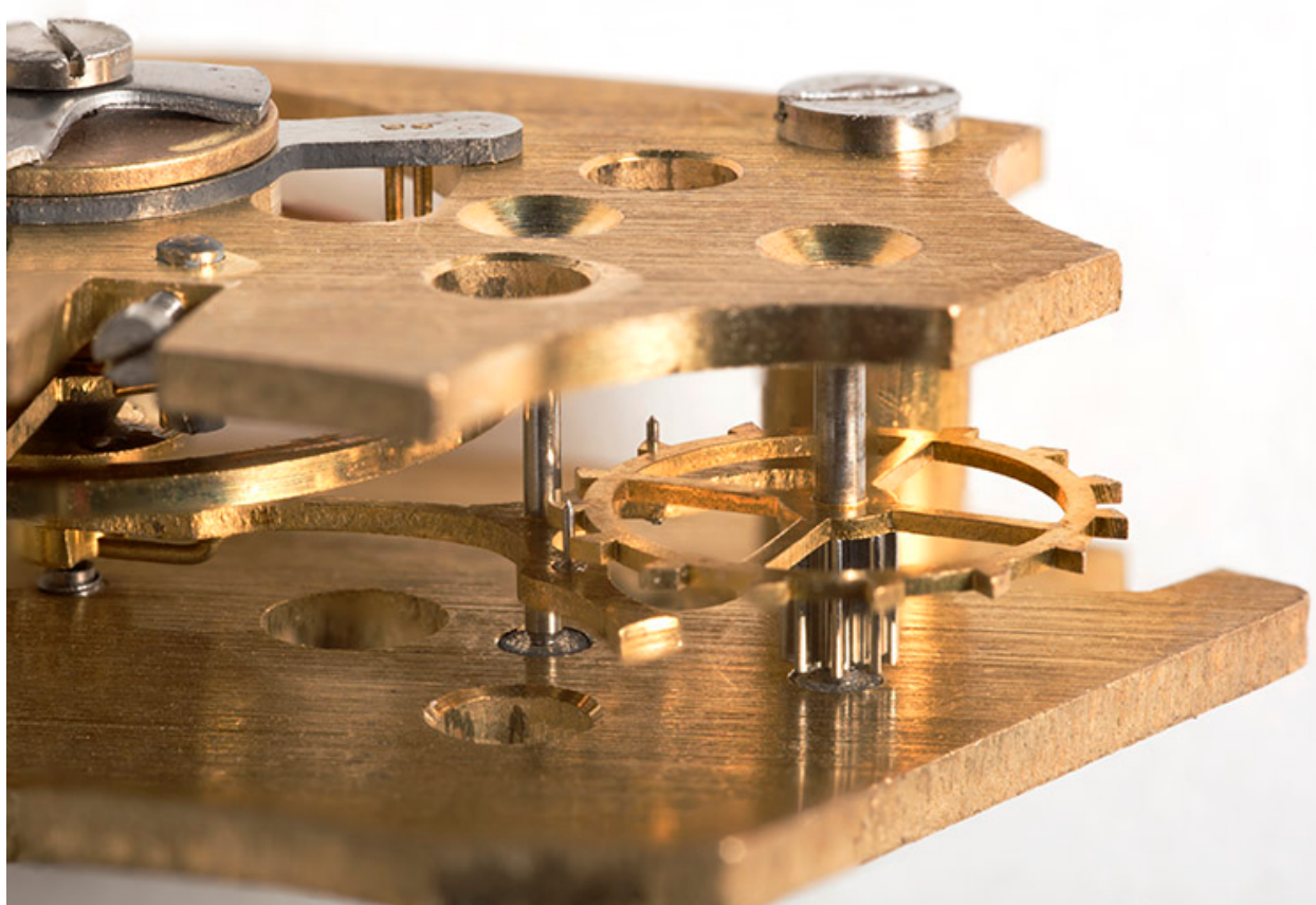
Echappement à chevilles : ancre et ses deux chevilles au centre, roue d'ancre à droite.
