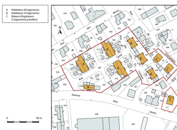
Plan-masse et de situation. Dess. Mathias Papigny IVR43_20132502543NUDA
