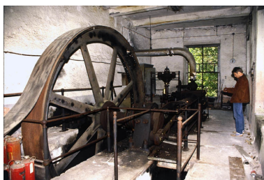
Vue d'ensemble de la salle des machines avec sa machine à vapeur. Phot. Yves Sancey IVR43_19999000226ZA
