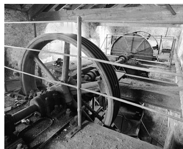
Roue de transmission de la machine à vapeur. Cette roue à 4 gorges est également couplée au volant d'inertie de la turbine (au second plan). Phot. Yves Sancey IVR43_19999000242X
