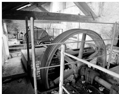
Roue de transmission et volant d'inertie de la turbine. Phot. Yves Sancey IVR43_19999000241X
