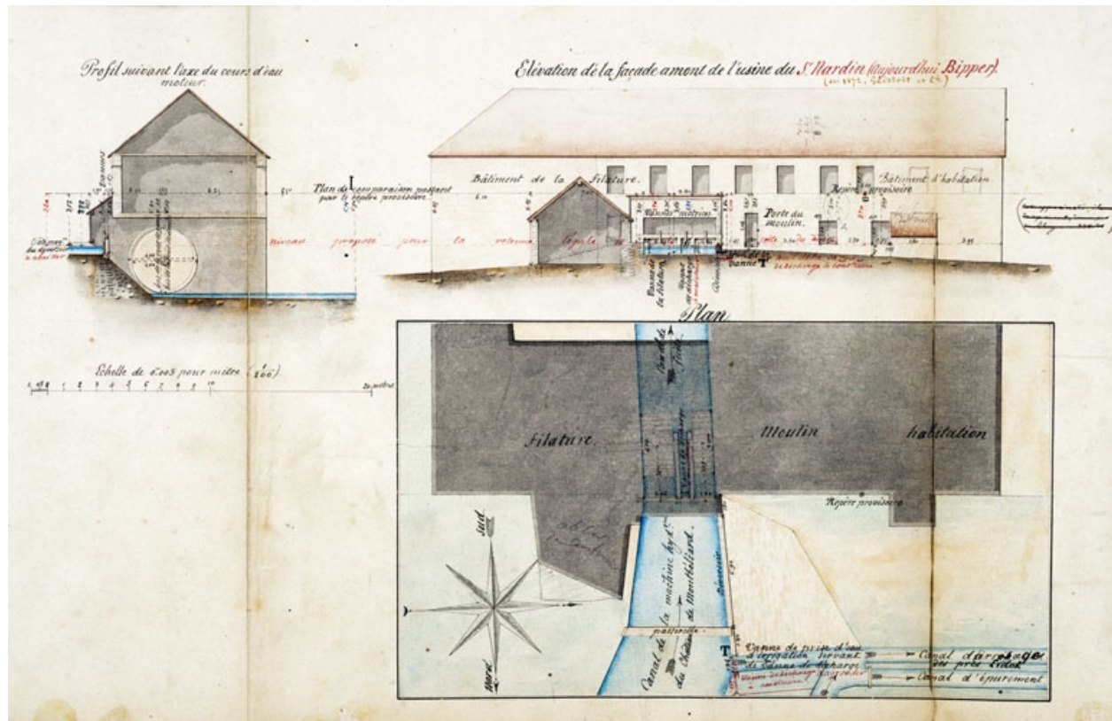
Règlement d'eau de l'usine du sieur Bipper [...]. Plan (plume, lavis), 1858, échelle 1/100.
