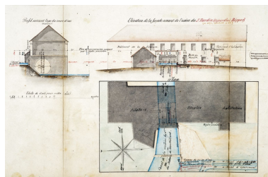
Règlement d'eau de l'usine du sieur Bipper [...]. Plan (plume, lavis), 1858, échelle 1/100. Phot. Jérôme Mongreville IVR43_20112500304NUC4A
