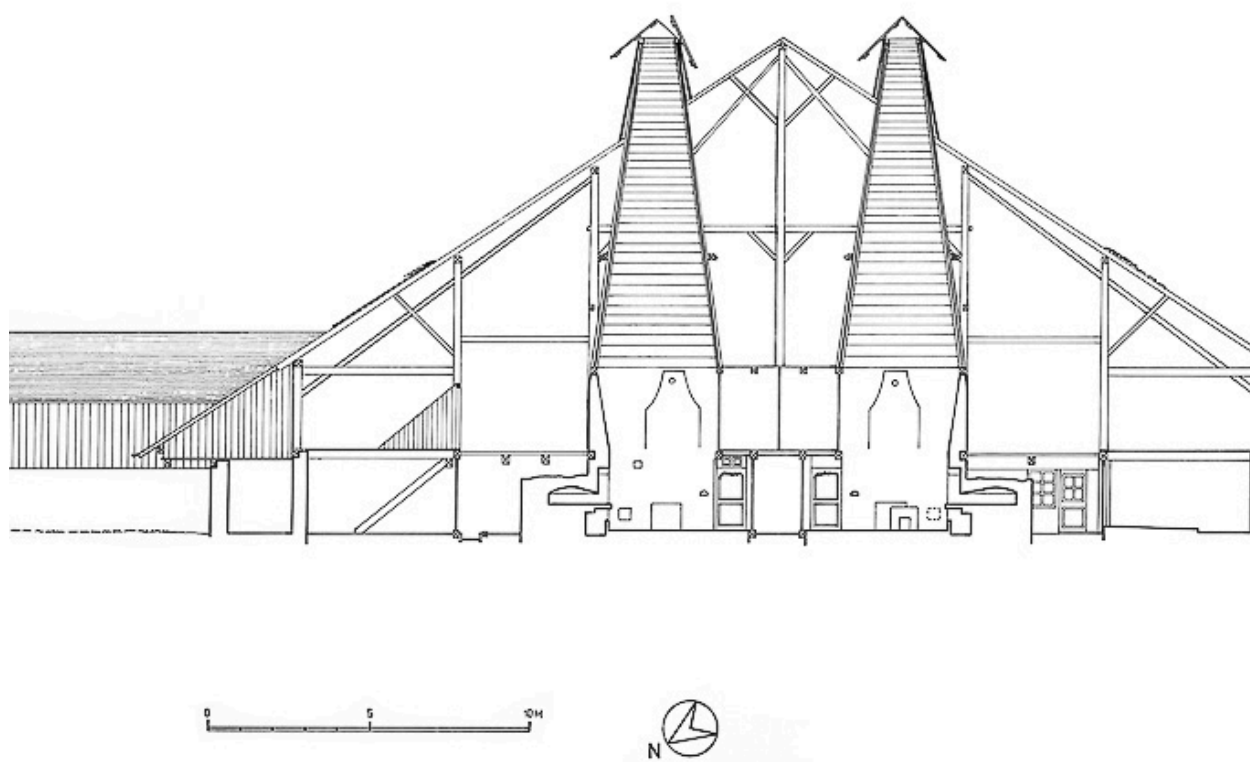
Coupe transversale.
