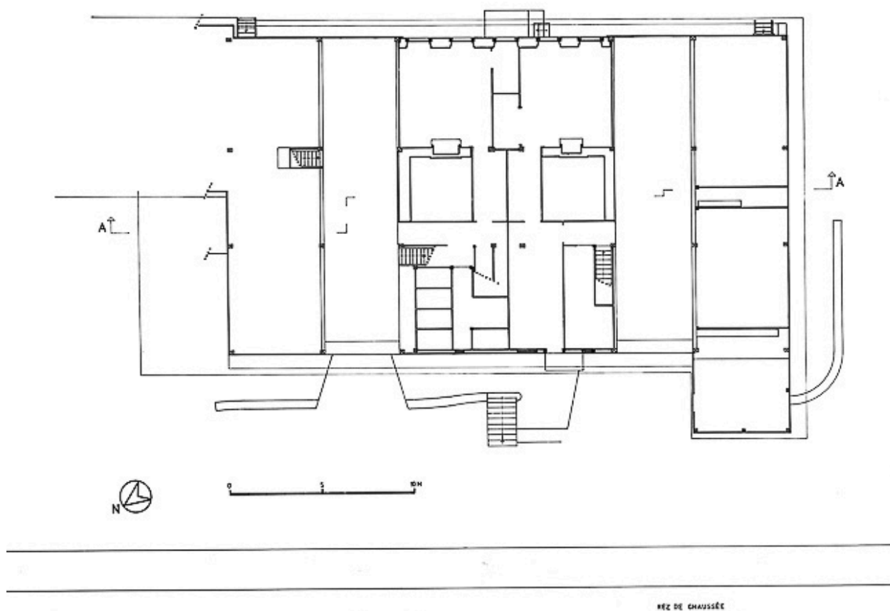
Plan au niveau du grenier.
