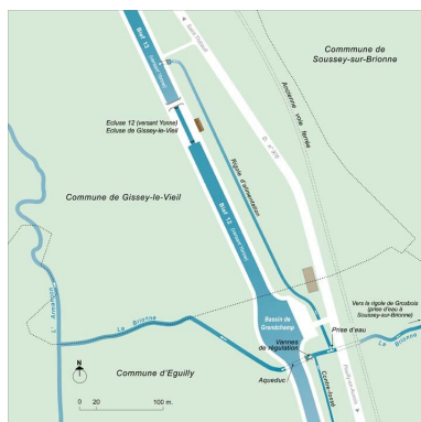
Plan schématique du réseau hydraulique aux biefs 12 et 13 du versant Yonne. Dess. Alain Morelière IVR26_20132100095NUDA
