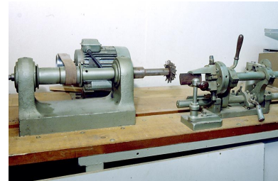
Machine à fraiser dite machine à arrondir. Phot. Jérôme Mongreville IVR43_20003901131ZA
