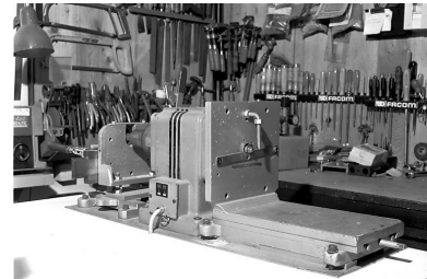
Machine à fraiser (fraiseuse- rainureuse) dite machine à chanfreiner et à faire les emplacements de charnière. Phot. Jérôme Mongreville IVR43_20003901118X
