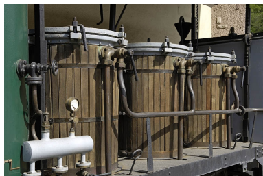
Récipients de l'alambic ambulant. Phot. Jérôme Mongreville IVR43_20057000376NUCA
