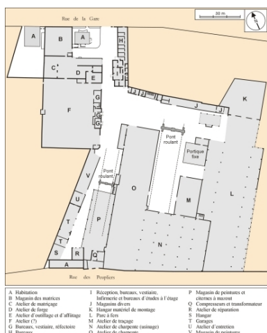
Plan-masse de l'usine en 1964. D'après un plan conservé dans les archives privées de l'entreprise, daté mai 1964, mis au net par A. Céréza. Dess. André Céréza IVR43_20057000167NUDA
