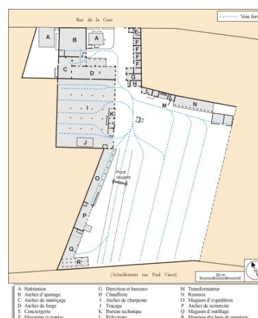
Plan-masse de l'usine en 1913. D'après un plan conservé dans les archives privées de l'entreprise, daté octobre 1913, mis au net par A. Céréza.
