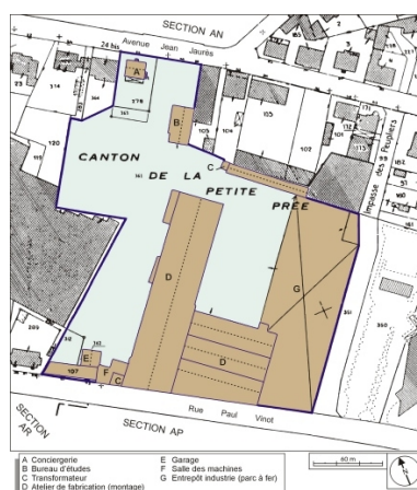
Plan-masse et de situation. Extrait du plan cadastral numérisé, 2005, section AO, 1:1000 réduit à 1:2000.
