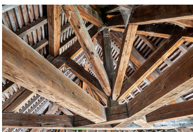
Charpente. Détail de l'enrayure sud. Phot. Jérôme Mongreville IVR43_20233900238NUC4A
