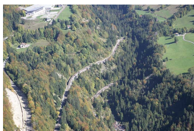
Viaduc de Romand (voie ferrée Andelot - La Cluse). Phot. Jean-Pierre Bévalot IVR43_20053901003NUCA
