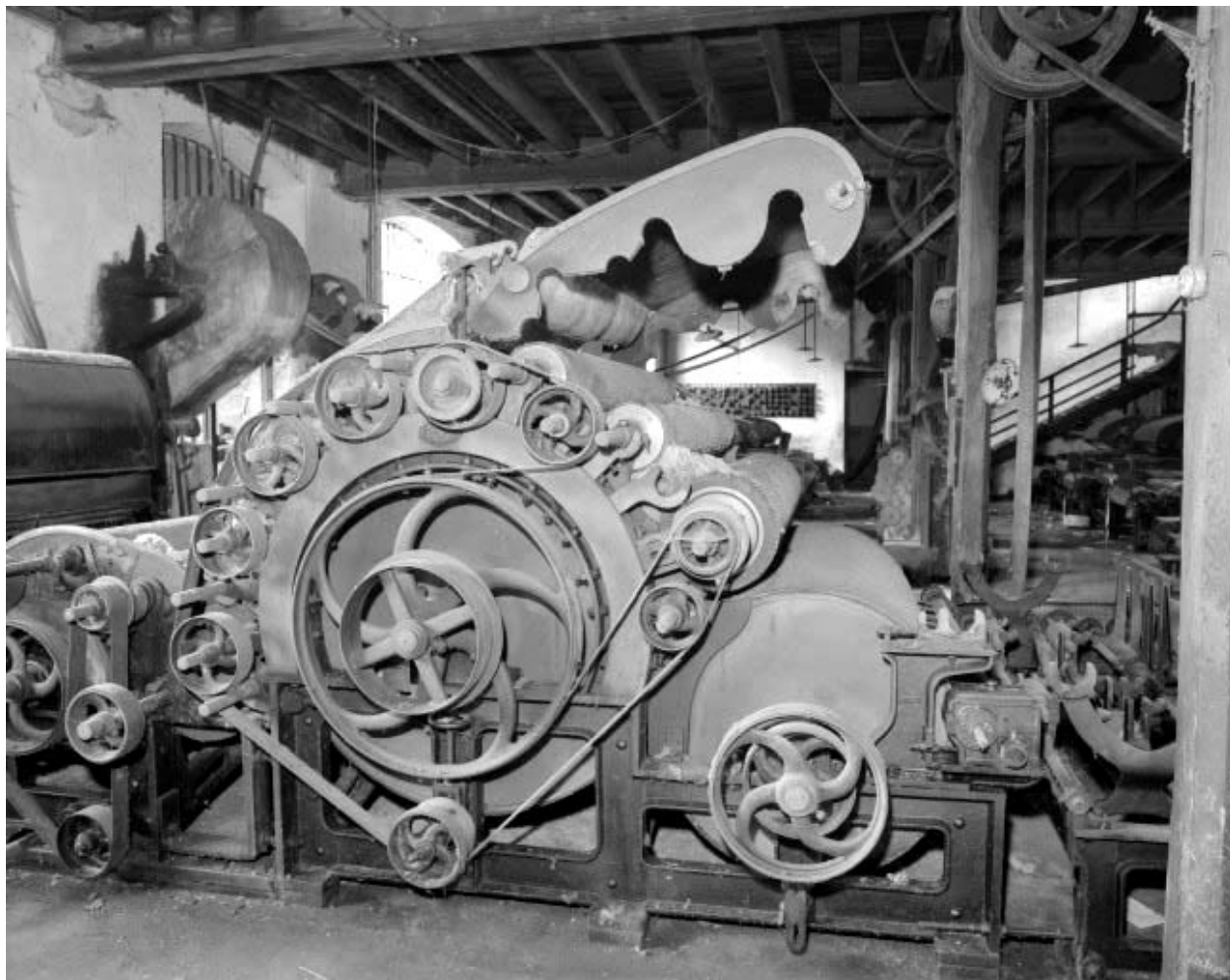
Grand tambour et cylindre peigneur.
