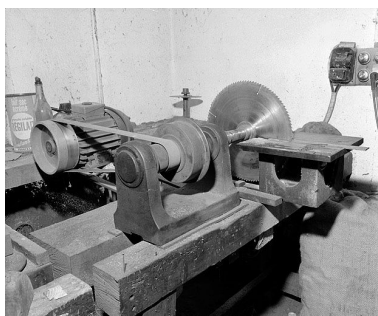
Vue d'ensemble de la scie de droite, servant au franchissage (mise à longueur). Phot. Jérôme Mongreville IVR43_20003901047X
