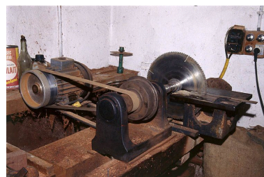
Vue d'ensemble de la scie de droite, servant au franchissage (mise à longueur). Phot. Jérôme Mongreville IVR43_20003901048ZA
