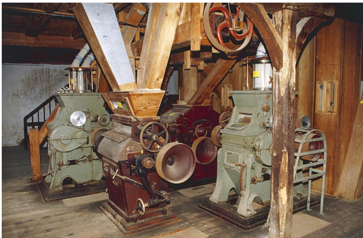
Appareils à cylindres (broyeurs et convertisseurs) au premier étage.
