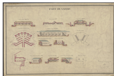
Fort de Varois [caponnière du front de tête, caponnière de gauche, plan des chapes]. 1887. Phot. Petot Frédéric, Autr. Biliette IVR26_20252100196NUC4A
