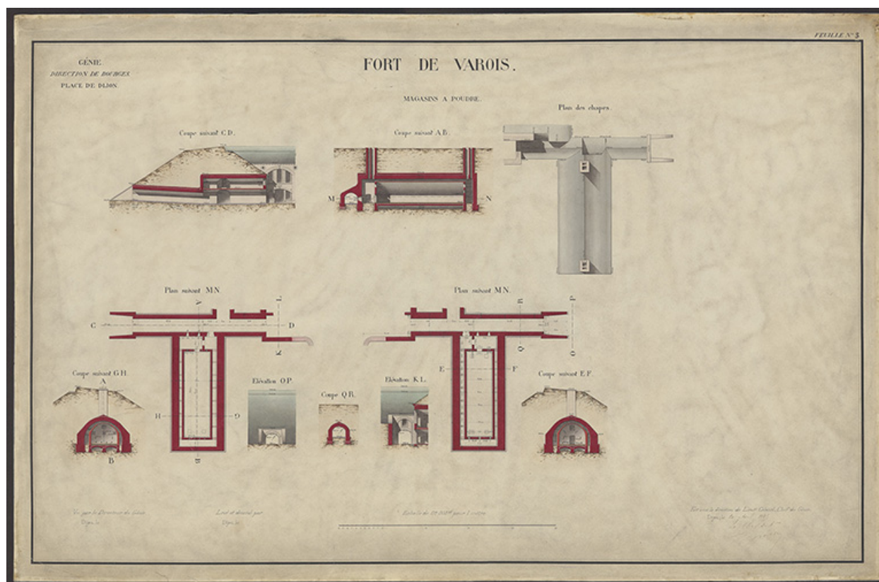
Forts de Varois. Magasins à poudre. 1885.
