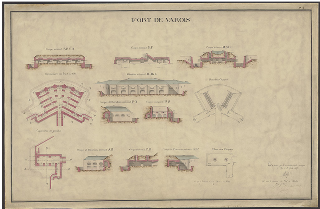
Fort de Varois [caponnière du front de tête, caponnière de gauche, plan des chapes]. 1887.
