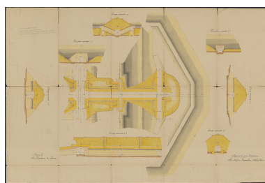
[Fort de Varois. Plans et coupes de la descente vers la double caponnière et de la traverse 17]. 1878.
