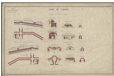
Fort de Varois. Descente de l'aileron de droite. 1885. Phot. Petot Frédéric, Autr. auteur inconnu IVR26_20252100199NUC4A
