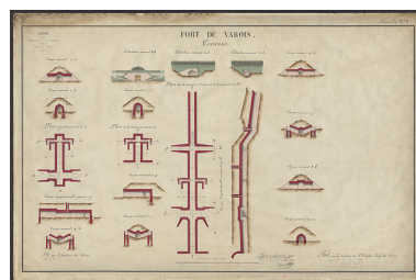
Fort de Varois. Traverses. 1880. Phot. Petot Frédéric, Autr. Gustave Nicolas Lamiable IVR26_20252100197NUC4A
