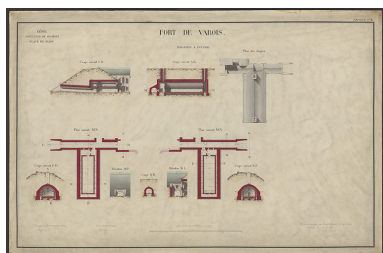
Forts de Varois. Magasins à poudre. 1885. Phot. Petot Frédéric, Autr. auteur inconnu IVR26_20252100198NUC4A
