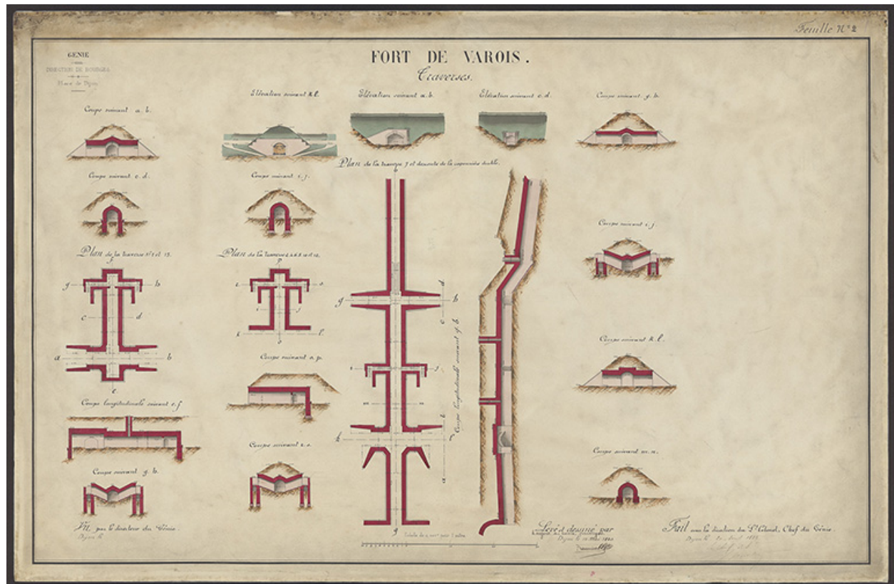
Fort de Varois. Traverses. 1880.
