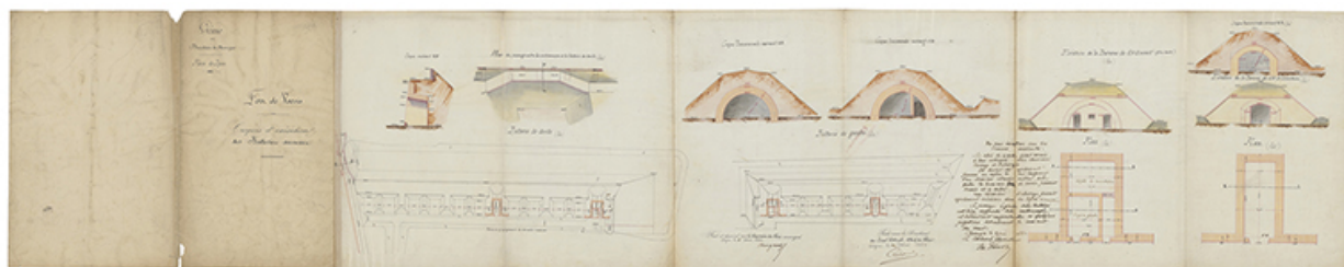
Fort de Varois. Croquis d'exécution des batteries annexes. 1880.
