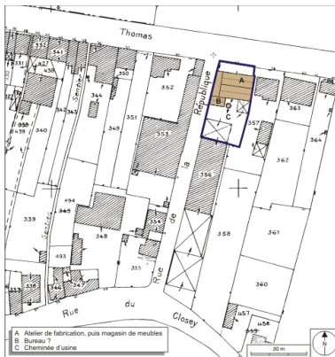
Plan-masse et de situation. Extrait du plan cadastral, 2008, section AI, 1:1000. Source : Direction générale des Finances Publiques - Cadastre ; mise à jour : 2008. Dess. André Céréza IVR43_20087000200NUDA
