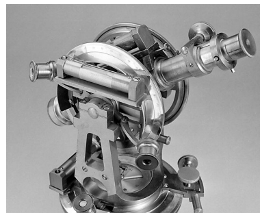
Vue plongeante sur la lunette et ses cercles. Phot. Jérôme Mongreville IVR43_20023900185X
