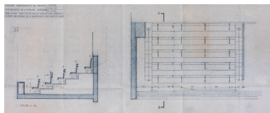
Plan et coupe des bancs de la tribune disposés en gradin. Phot. Pierre-Marie Barbe-Richaud, Autr. Oskar Bitterli, Autr. Barnabé Augros IVR26_20227100256NUC2A
