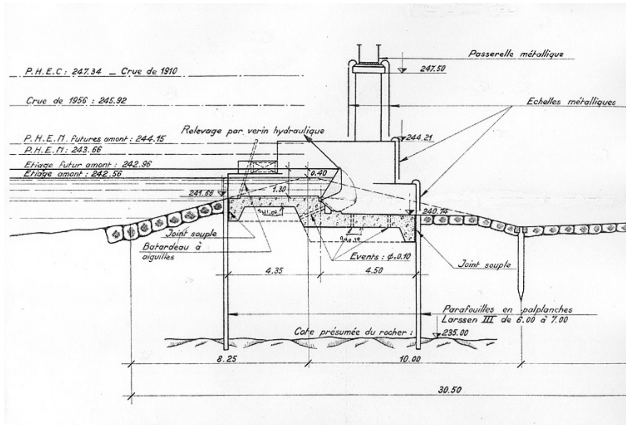
Barrage de la Malate. Equipement avec bouchure mobile. Coupe transversale du barrage (partie mobile), 1959.
