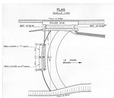
Barrage de la Malate. Equipement avec bouchure mobile. Plan, 1959. Phot. Yves Sancey, Phot. Escoffier IVR43_20062500419NUCA
