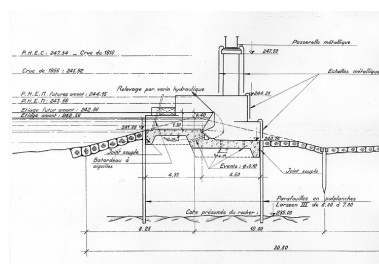
Barrage de la Malate. Equipement avec bouchure mobile. Coupe transversale du barrage (partie mobile), 1959. Phot. Yves Sancey, Phot. Escoffier IVR43_20062500420NUCA
