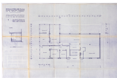
Schwartzmann Frères [...] Projet d'extension des magasins et bureaux. 2. Plan du rez de chaussée [et coupe], 24 février 1966. Phot. Sonia Dourlot, Autr. Jean Arbaret IVR43_20182500183NUC4A
