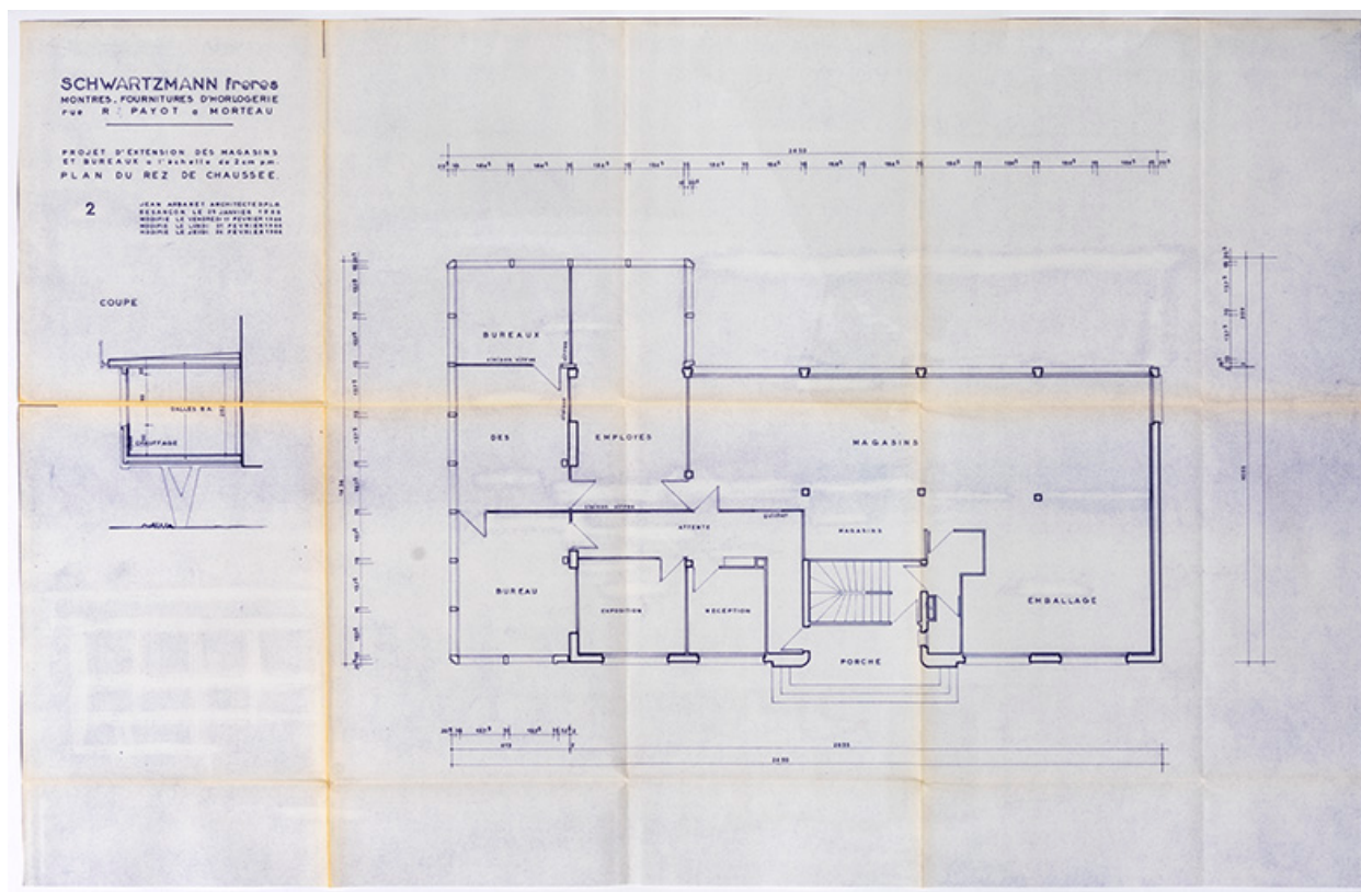
Schwartzmann Frères [...] Projet d'extension des magasins et bureaux. 2. Plan du rez de chaussée [et coupe], 24 février 1966.
