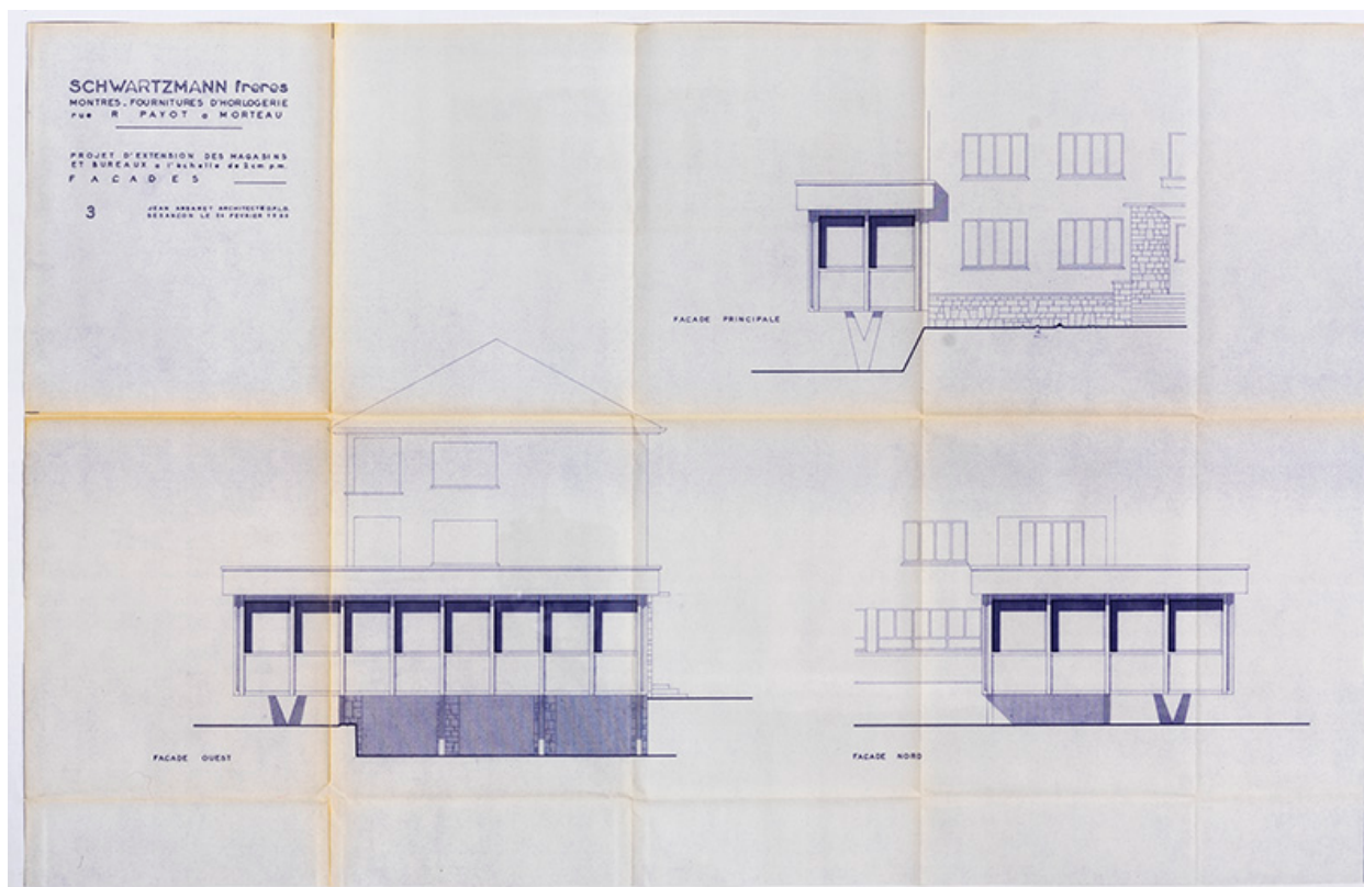
Schwartzmann Frères [...] Projet d'extension des magasins et bureaux. 3. Façades, 24 février 1966.
