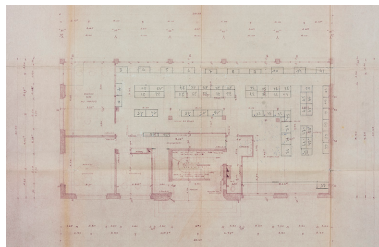
Schwartzmann Frères [...] Projet de construction de magasins, bureaux, logements. Plan du Rez- de-chaussée, 14 novembre 1952. Phot. Sonia Dourlot, Autr. Jean Arbaret IVR43_20182500185NUC4A
