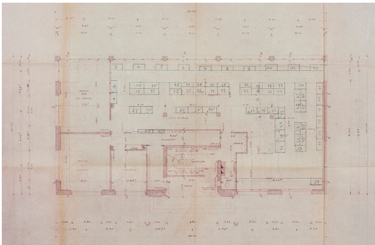
Schwartzmann Frères [...] Projet de construction de magasins, bureaux, logements. Plan du Rez-de-chaussée, 14 novembre 1952.
