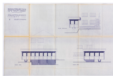
Schwartzmann Frères [...] Projet d'extension des magasins et bureaux. 3. Façades, 24 février 1966. Phot. Sonia Dourlot, Autr. Jean Arbaret IVR43_20182500184NUC4A
