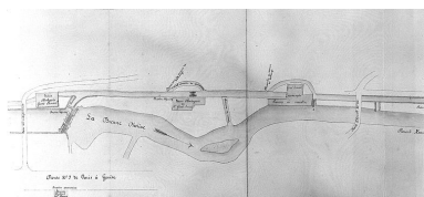
Projet de révision du règlement hydraulique des usines Girod Emmanuel, Prost Frères et Bonnefoy Valère [détail de la partie gauche : rue Pierre Morel], 1863. Plan des lieux et dessins de détail (détail de la partie gauche) Phot. Jérôme Mongreville, Autr. Antoine IVR43_19993900504V
