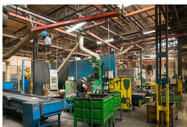
Atelier de parachèvement (2). Phot. Jérôme Mongreville IVR43_20132500986NUC4A
