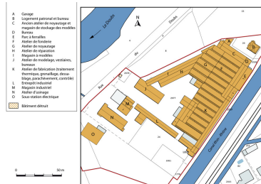
Plan-masse et de situation. Extrait du plan cadastral numérisé, section C, échelle 1:1250. Dess. Mathias Papigny IVR43_20142500572NUDA
