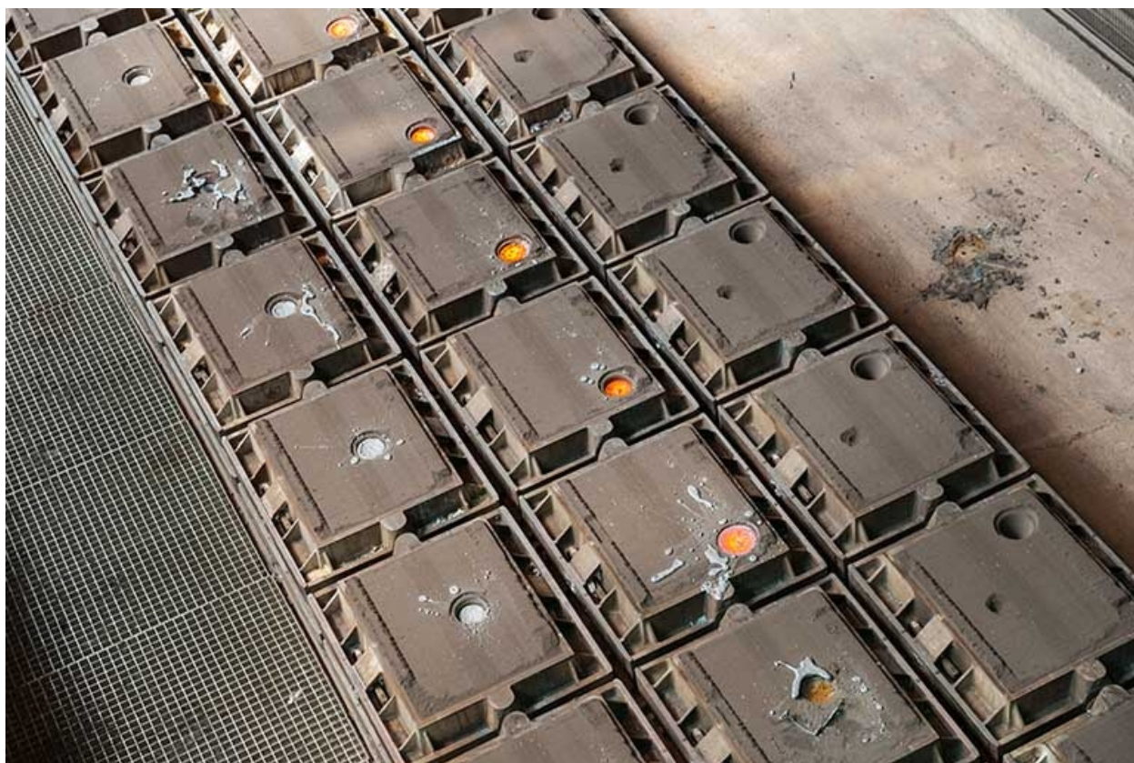
Ligne de moulage. Détail des moules (2).
