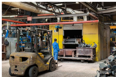
Décocheuse (1).
