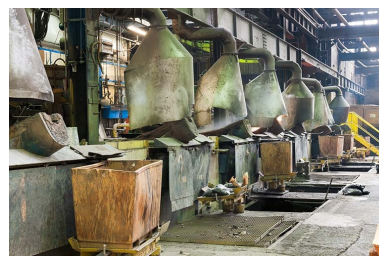
Batterie de fours à induction (1). Phot. Jérôme Mongreville IVR43_20132500948NUC4A
