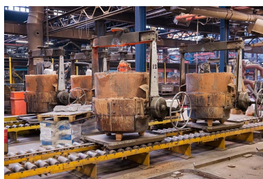
Poches de coulée avant réfection (2).
