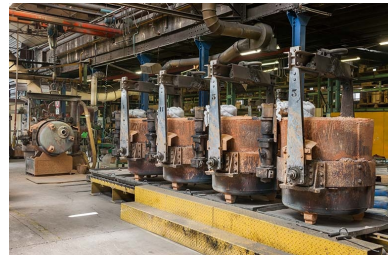
Poches de coulée avant réfection (1). Phot. Jérôme Mongreville IVR43_20132500966NUC4A
