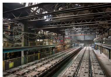
Ligne de moulage. Vue d'ensemble.
