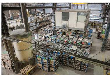
Aire de stockage des modèles et des noyaux (1). Phot. Jérôme Mongreville IVR43_20132500972NUC4A
