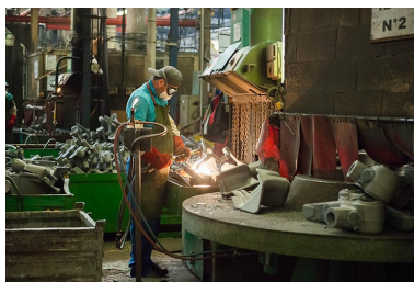
Découpage de pièces au chalumeau (1).
