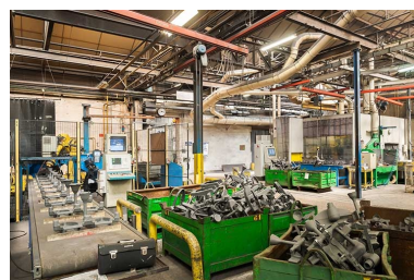
Atelier de parachèvement. Ligne robotisée. Phot. Jérôme Mongreville IVR43_20132500987NUC4A
