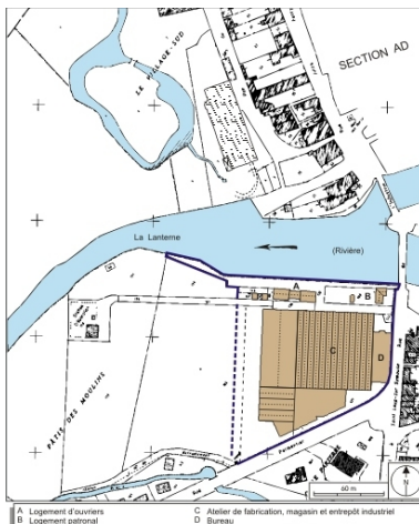
Plan-masse et de situation. Extrait du plan cadastral numérisé, 2008, section B, 1:1250 réduit à 1:2000. Source : Direction générale des Finances Publiques - Cadastre ; mise à jour : 2008. Dess. André Céréza IVR43_20087000196NUDA
