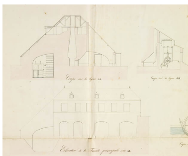
Plan, coupes et élévation du fourneau et des patouillets de Renaucourt [...] [coupe et élévation de la façade principale].
