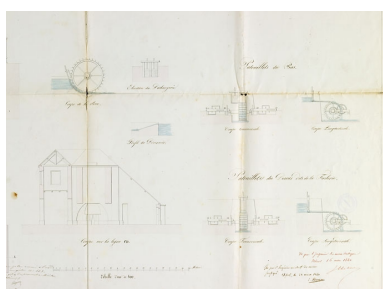
Plan, coupes et élévation du fourneau et des patouillets de Renaucourt [...] [coupe du haut fourneau et des patouillets].
