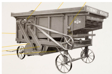
Batteuse Estienney-Ménétrier 140 SAB.
