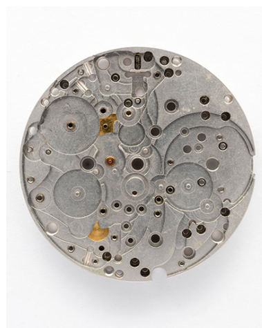
Platine, face côté cadran. Phot. Sonia Dourlot IVR43_20182501176NUC4A
