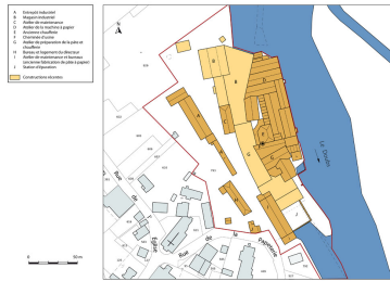
Plan-masse et de situation. Dess. Mathias Papigny IVR43_20132502684NUDA
