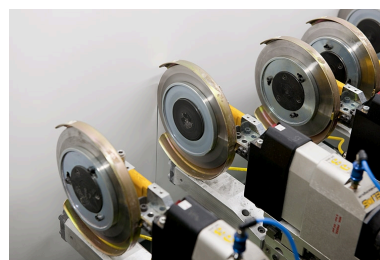
Têtes de découpage. Phot. Jérôme Mongreville IVR43_20122500990NUC4A
