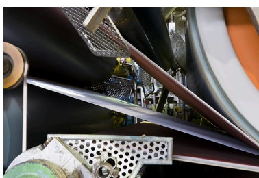
Passage de la feuille de papier entre les cylindres de pressage et d'égouttage. Vue de face. Phot. Jérôme Mongreville IVR43_20122500982NUC4A
