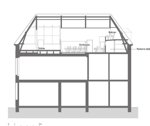
Coupe longitudinale schématique du bâtiment. Dess. Aline Thomas IVR26_20238901023NUDA
