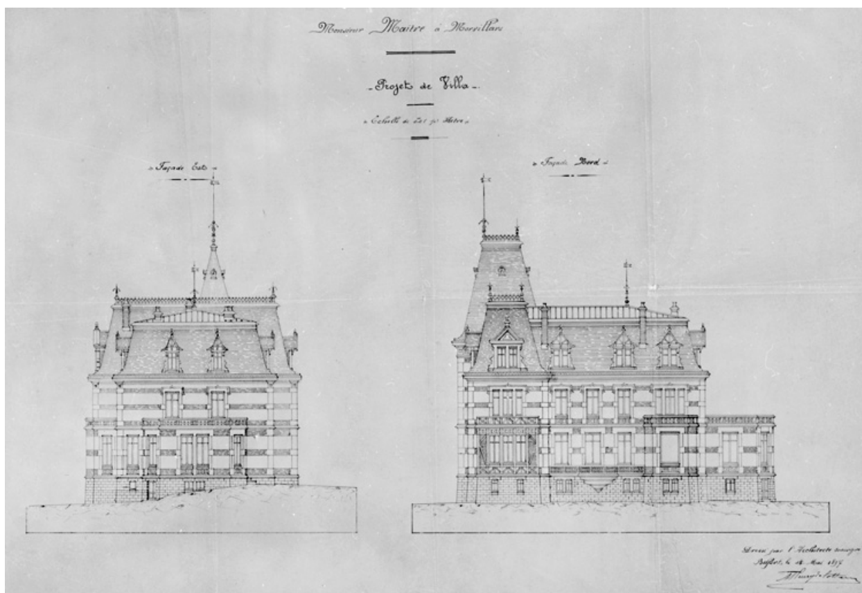
Monsieur Maître à Morvillars. Projet de villa. Façade est et façade nord.
