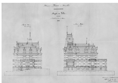
Monsieur Maître à Morvillars. Projet de villa. Façade est et façade nord. Phot. Jérôme Mongreville, Phot. Anthime Fleury de la Hussinière IVR43_20019000015V
