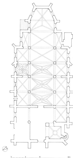
Plan. Dess. Alain Morelière
