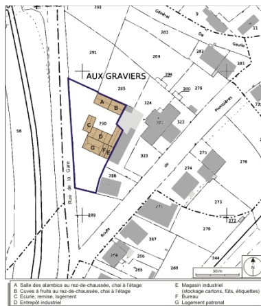
Plan-masse et de situation. Extrait du plan cadastral numérisé, 2008, section AE, 1:1000. Source : Direction générale des Finances Publiques - Cadastre ; mise à jour : 2008. Dess. André Céréza IVR43_20087000217NUDA
