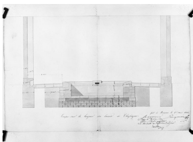
Coupe transversale du lavoir, devis daté du 1er mai 1836 par Champonnois aîné (architecte). Phot. Jean-Luc Duthu, Autr. Champonnois aîné (architecte) IVR26_19802101653V
