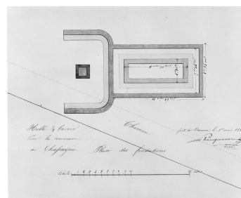
Plan des fondations du lavoir, devis daté du 1er mai 1836 par Champonnois aîné (architecte). Phot. Jean-Luc Duthu, Autr. Champonnois aîné (architecte) IVR26_19802101652V
