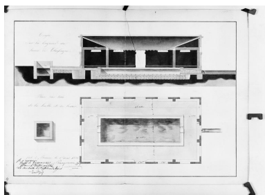
Plan et coupe longitudinale, devis daté du 1er mai 1836 par Champonnois aîné (architecte). Phot. Jean-Luc Duthu, Autr. Champonnois aîné (architecte) IVR26_19802101650V
