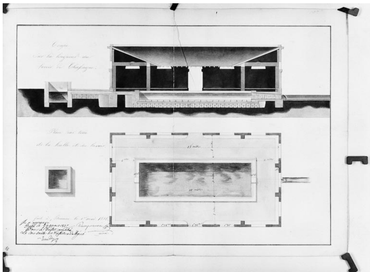
Plan et coupe longitudinale, devis daté du 1er mai 1836 par Champonnois aîné (architecte).
