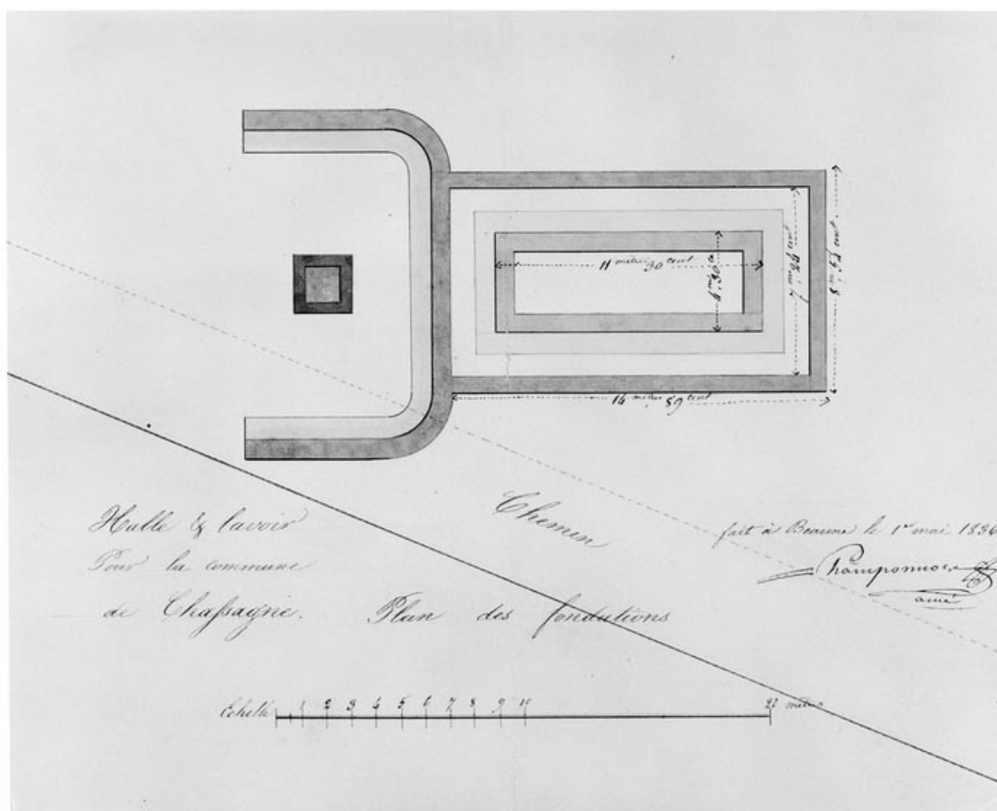
Plan des fondations du lavoir, devis daté du 1er mai 1836 par Champonnois aîné (architecte).
