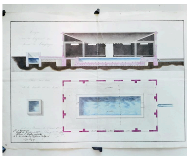
Plan et coupe longitudinale, devis daté du 1er mai 1836 par Champonnois aîné (architecte). Phot. Michel Thierry, Autr. Champonnois aîné (architecte) IVR26_19812100307XE
