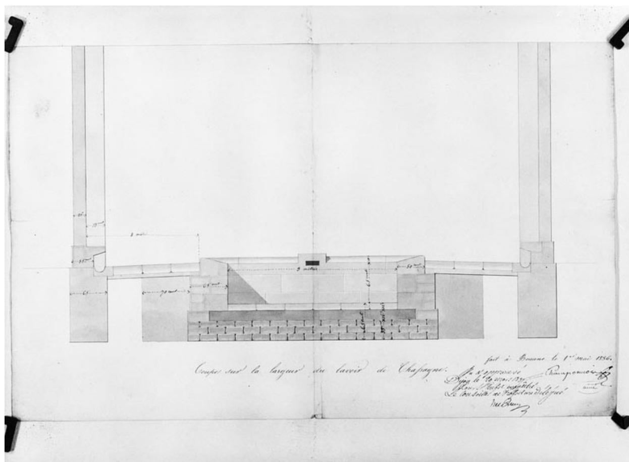
Coupe transversale du lavoir, devis daté du 1er mai 1836 par Champonnois aîné (architecte).
