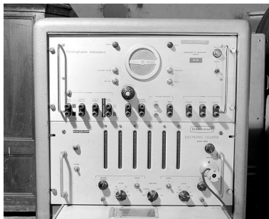
Chronographe totalisateur Ebauches et compteur électronique Beckman.
