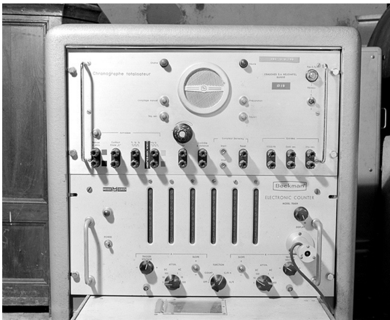
Chronographe totalisateur Ebauches et compteur électronique Beckman.
