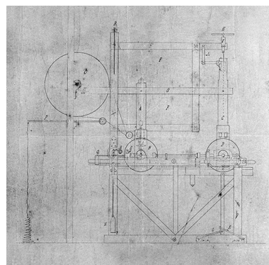
Elévation de la face latérale gauche. Phot. Jérôme Mongreville IVR43_20003901203V
