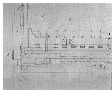
Elévation de la face postérieure : détail de la partie gauche du plan. Phot. Jérôme Mongreville IVR43_20003900949X
