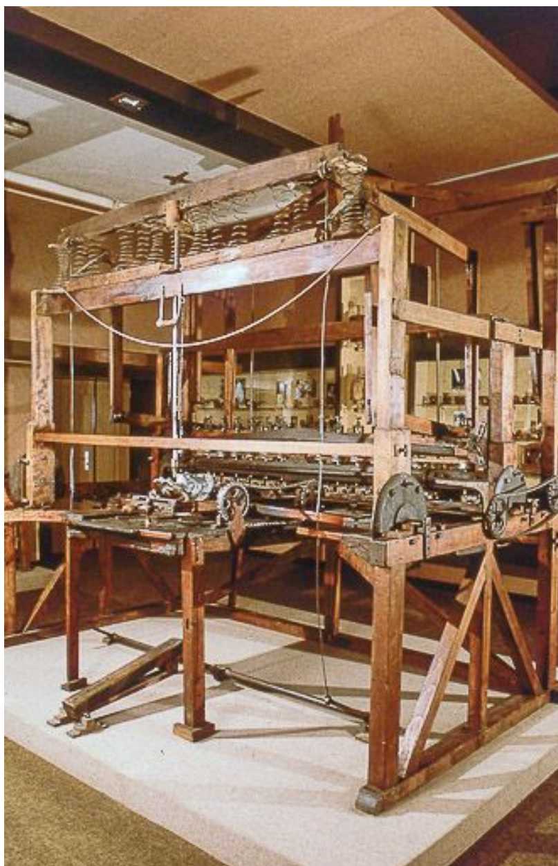
Vue d'ensemble de trois quarts droite.
