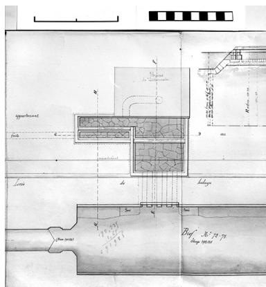
Dessin d'une usine pour filature à laines et foulons [...]. Phot. Yves Sancey, Autr. H. Bastien IVR43_19903901034X
