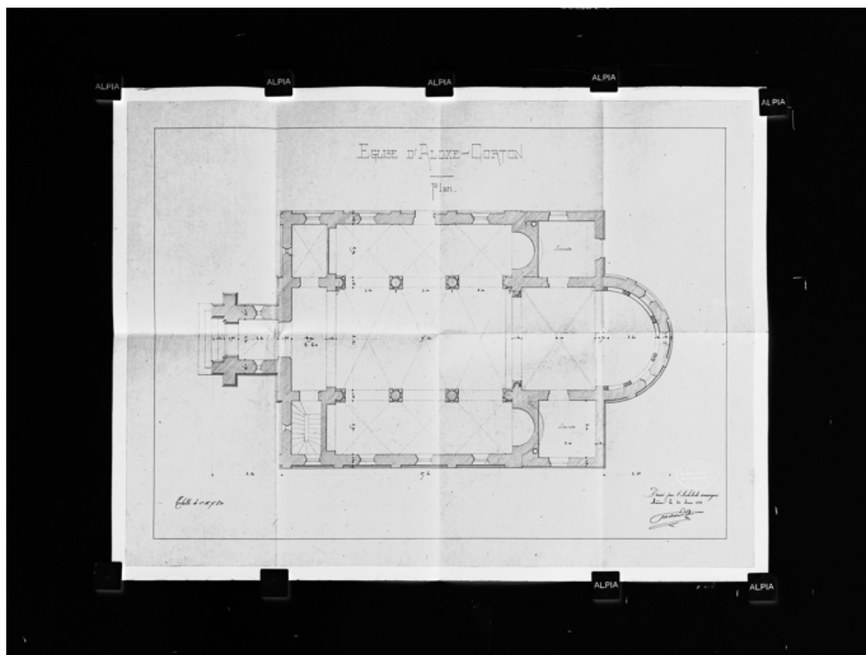
Plan de l'église d'Aloxe-Corton, dressé par l'architecte Pinchard le 30 juin 1888 (Archives communales, Aloxe-Corton).
