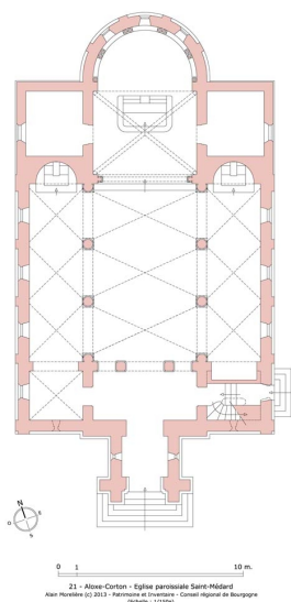
Plan de l'église. Dess. Alain Morelière IVR26_20132101070NUDA
