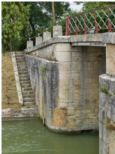
Vue des piles du pont. Phot. Pierre-Marie Barbe-Richaud IVR26_20178900069NUC2A
