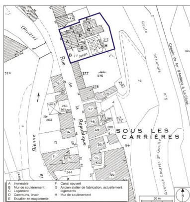
Plan-masse et de situation. Extrait du plan cadastral, 1980, section AD, échelle 1:1000. Dess. André Céréza IVR43_20093900259NUDA
