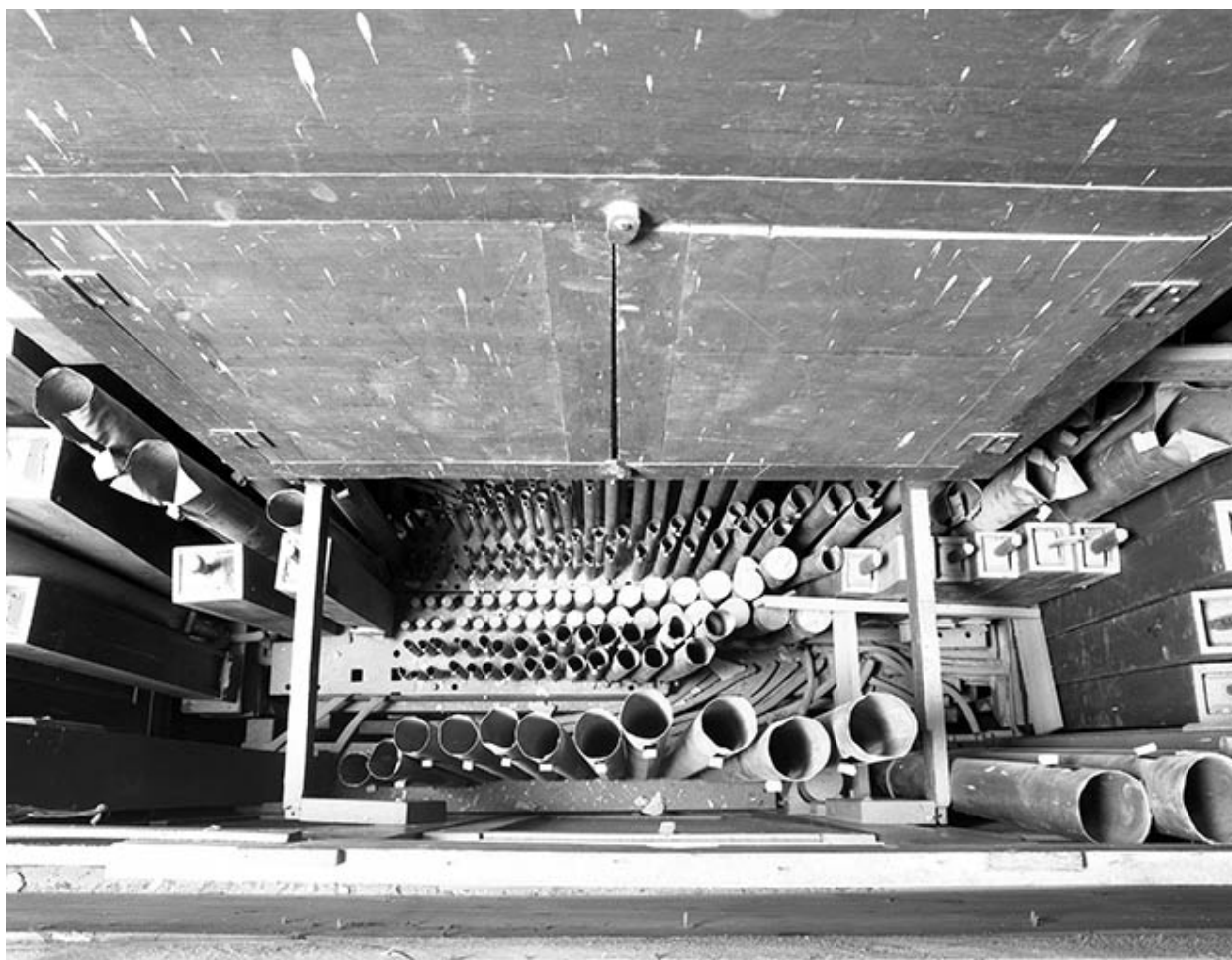
Vue plongeante sur la tuyauterie.
