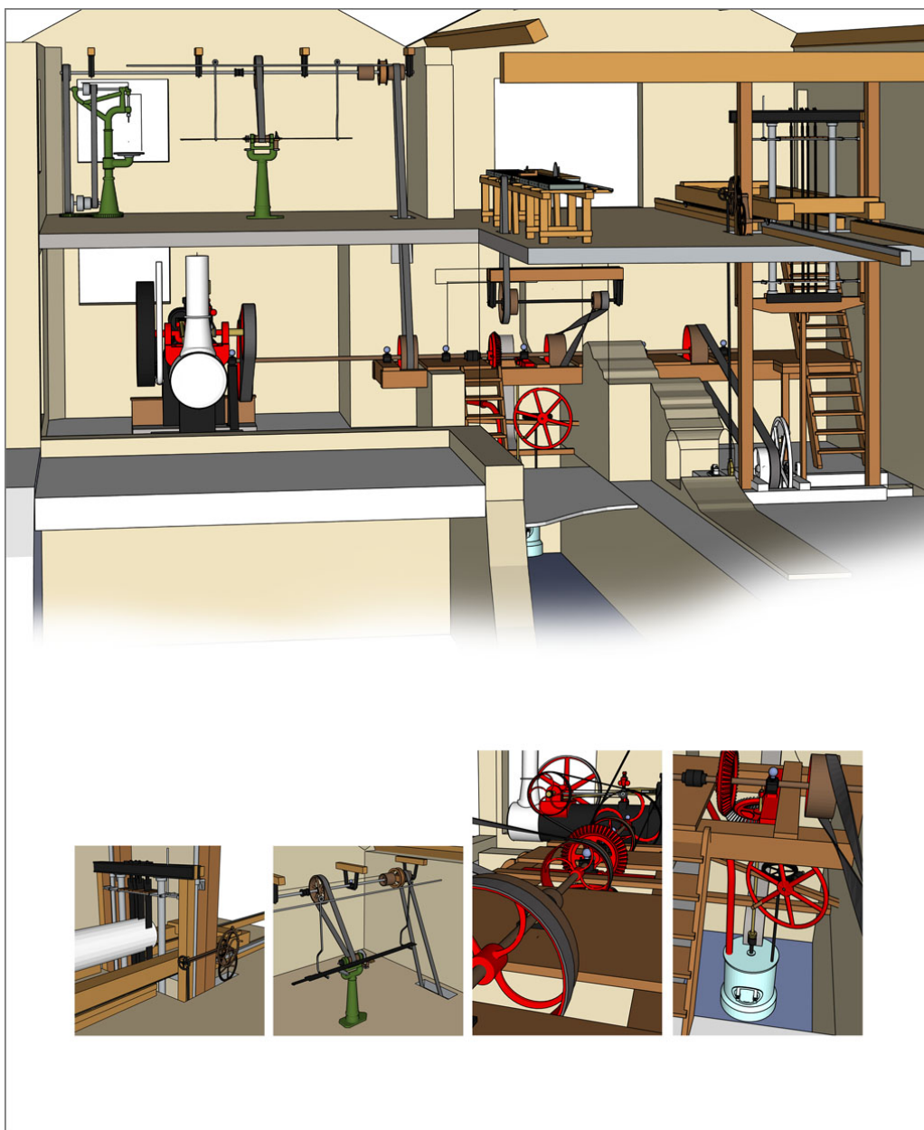
Schéma de distribution de la force motrice.
