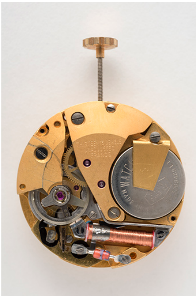
Mouvement de montre électromécanique Lip R 148, vu côté ponts.
