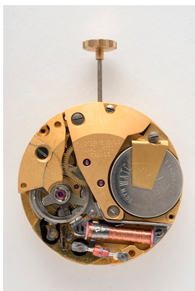
Mouvement de montre électromécanique Lip R 148, vu côté ponts. Phot. Sonia Dourlot IVR43_20152502569NUC4A
