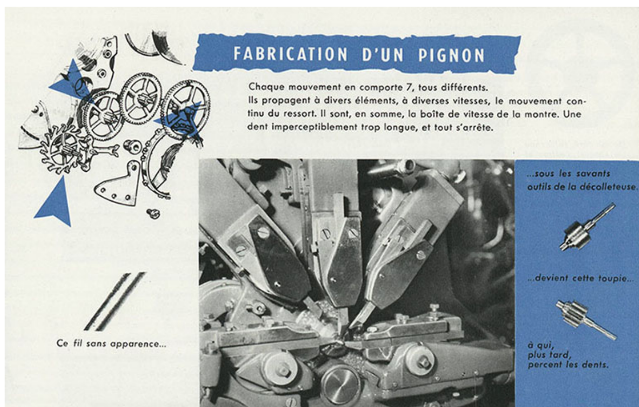
Fabrication d'un pignon, fotogr., 1956.
