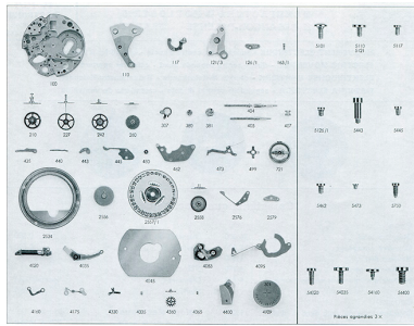
Montre-bracelet électromécanique dite Lip Electronic - R 184 Electrique [éclaté des fournitures], 1973. Autr. auteur inconnu IVR43_20162500115NUC4A
