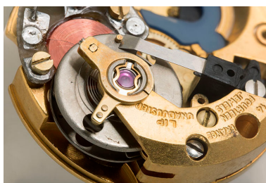
Mouvement Lip RE 50 : amortisseur Incabloc, balancier et bobine. Phot. Sonia Dourlot IVR43_20152502567NUC4A
