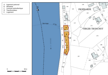
Plan-masse et de situation. Extrait du plan cadastral, 2015, section D. Dess. Mathias Papigny IVR43_20152502645NUDA
