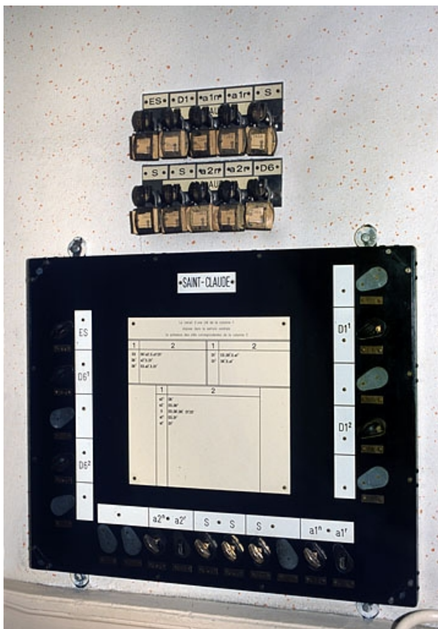
Serrure centrale à clefs S dans le bureau de l'agent de circulation (bâtiment des voyageurs).
