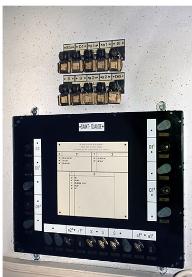
Serrure centrale à clefs S dans le bureau de l'agent de circulation (bâtiment des voyageurs). Phot. Yves Sancey IVR43_20053900809ZA
