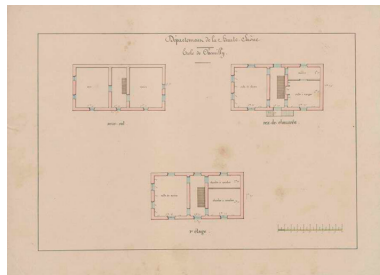
Plans en coupe du sous-sol, rez-de-chaussée et premier étage de l'école de Chemilly Phot. Jérôme Mongreville IVR43_20167001523NUC2A
