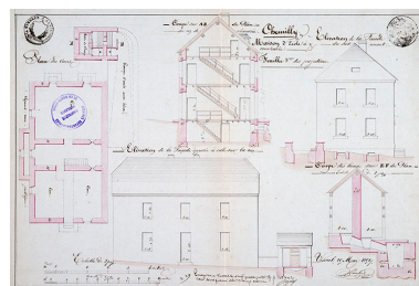
Plans de la maison d'école à construire, 1851 Phot. Jérôme Mongreville IVR43_20167001554NUC4A
