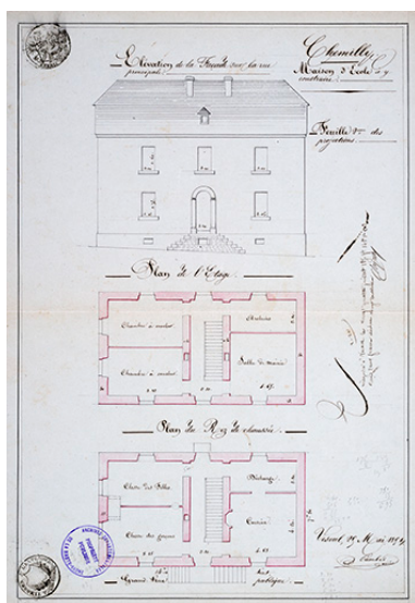
Plans de la façade sur rue de l'école à construire, 1851 Phot. Jérôme Mongreville IVR43_20167001555NUC4A
