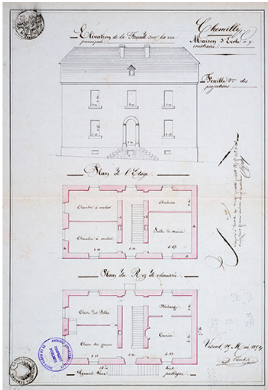
Plans de la façade sur rue de l'école à construire, 1851
