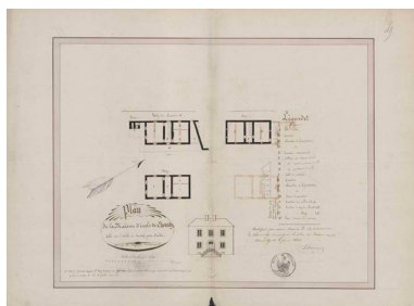
Plans de la maison d'école de Chemilly Phot. Jérôme Mongreville IVR43_20167001524NUC2A
