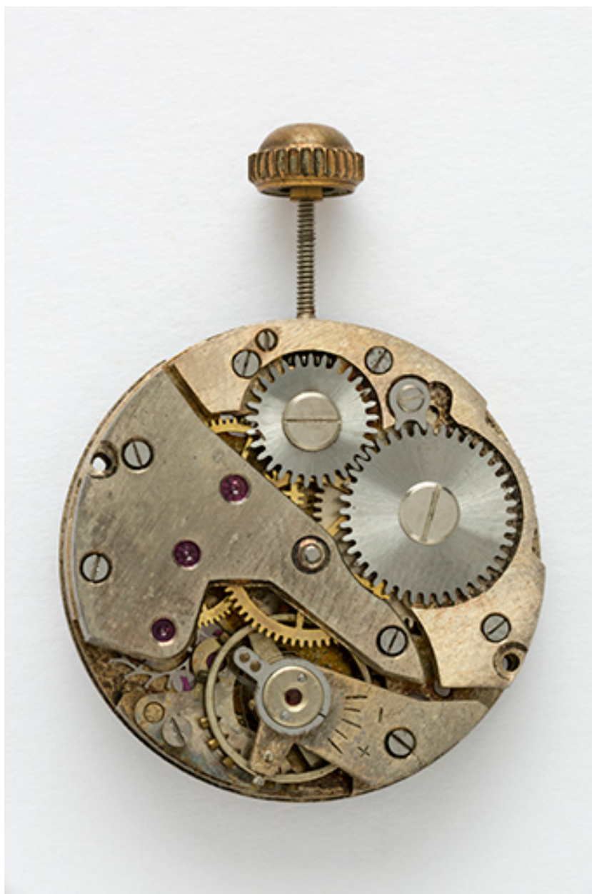
Mouvement Cupillard VC 233 : face côté ponts.
