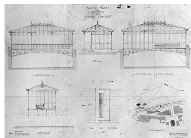
Construction d'un lavoir couvert [projet non réalisé de lavoir enjambant la Bienne], 1877. Phot. Jérôme Mongreville, Phot. Paillot IVR43_19953900063X
