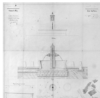
Commune de Morez. Projet d'une fontaine [place de la Samaritaine, actuellement Jules Girod], 1840. Phot. Jérôme Mongreville, Autr. Vital (architecte) NEPASUTILISER IVR43_19953900065X
