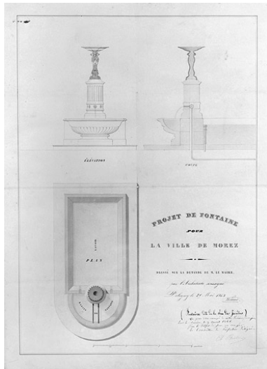
Projet de fontaine pour la ville de Morez (Fontaine dite de la Rue des Jardins) [projet non réalisé], 1843. Phot. Jérôme Mongreville, Phot. Narcisse Perrard IVR43_19953900027V
