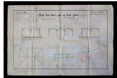
Projet d'une toiture pour un lavoir public (Quai de l'ancienne place), 1850. Phot. Yves Sancey, Phot. Vital Ponard IVR43_20103900067NUC2A
