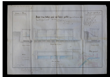
Projet d'une toiture pour un lavoir public (Rue des promenades), 1850. Phot. Yves Sancey, Phot. Vital Ponard IVR43_20103900066NUC2A
