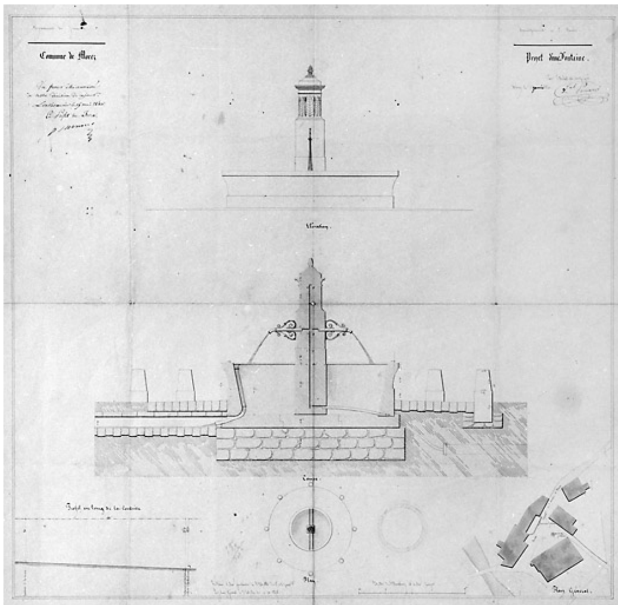
Commune de Morez. Projet d'une fontaine [place de la Samaritaine, actuellement Jules Girod], 1840.
