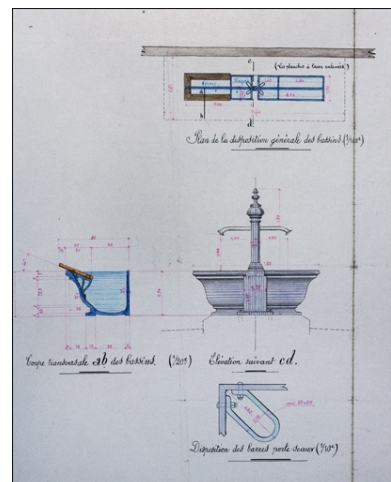
Etablissement de bassins en fonte au lavoir public dit de l'Hôpital. Dessins, 1912. Phot. Yves Sancey, Phot. Lacroix IVR43_20103900055NUC2A
