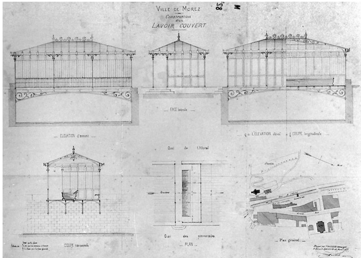
Construction d'un lavoir couvert [projet non réalisé de lavoir enjambant la Bienne], 1877.
