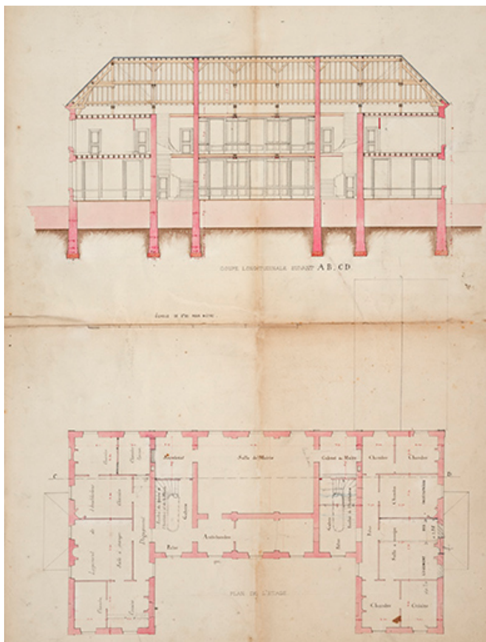
Renahy. Coupe longitudinale et plan de l'étage. 1866.
