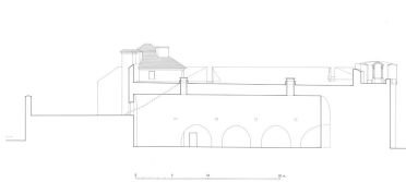
Grosse tour boulevard, improprement appelé bastion de l'Hôtel-Dieu : coupe transversale. Dess. Alain Morelière IVR26_20122100057A2YY
