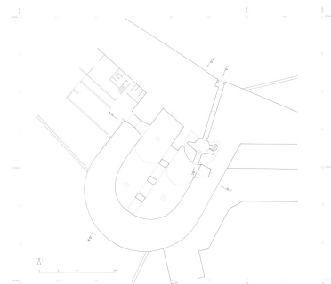
Grosse tour boulevard, improprement appelé bastion de l'Hôtel-Dieu : plan du niveau inférieur. Dess. Alain Morelière IVR26_20122100053A0YY
