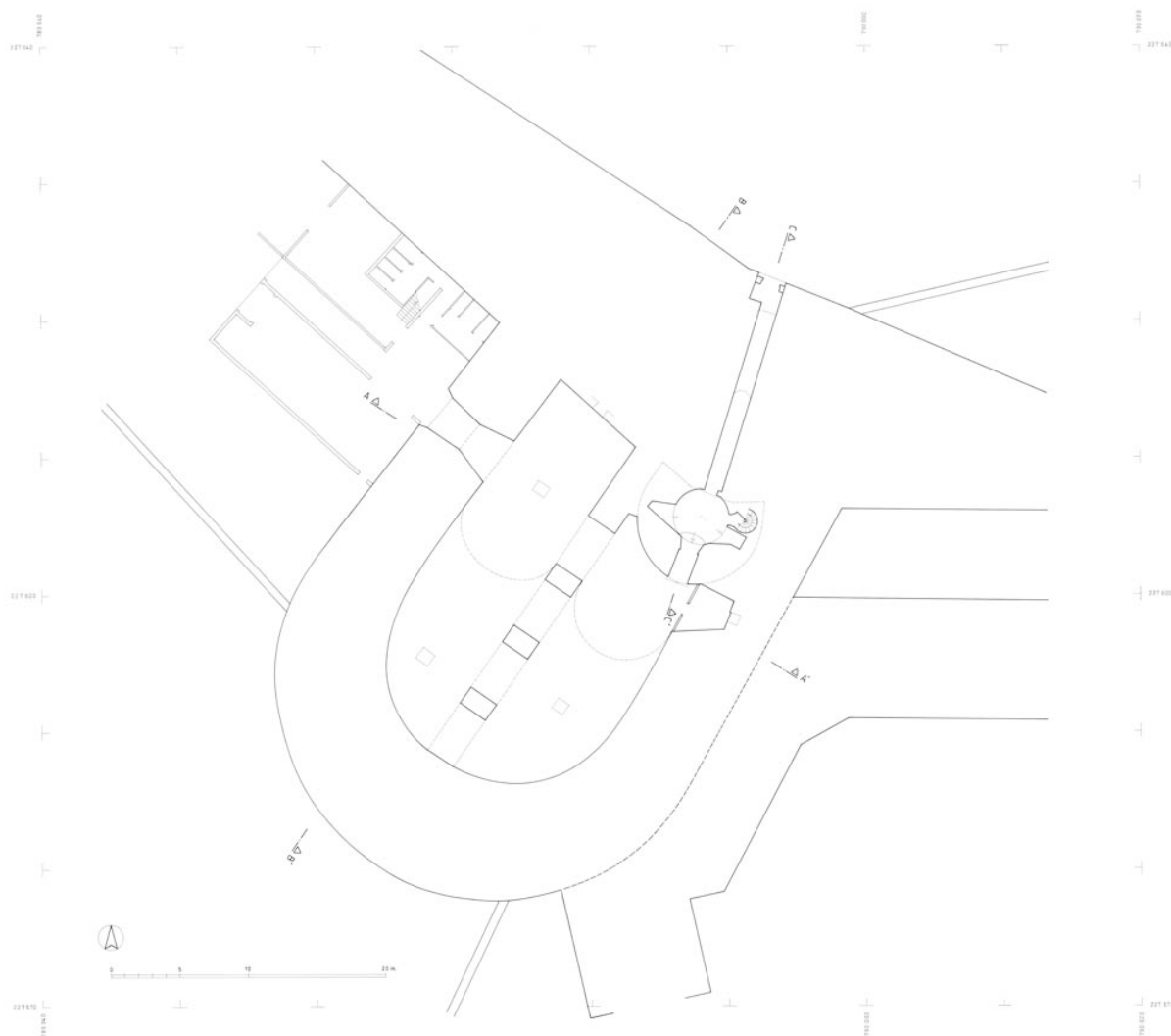
Grosse tour boulevard, improprement appelé bastion de l'Hôtel-Dieu : plan du niveau inférieur.
