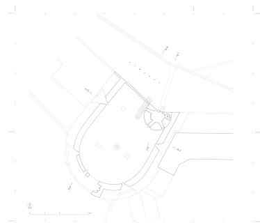
Plan sur terrasse du boulevard et du niveau supérieur de la tour des Cordeliers. Dess. Alain Morelière IVR26_20122100055A0YY
