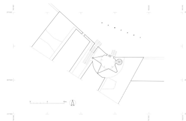
Plan du niveau intermédiaire. Dess. Alain Morelière IVR26_20122100054A2YY
