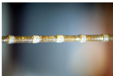
Scie à fil Ravet : détail du fil diamanté. Phot. Laurent Poupard IVR43_19933900462ZA
